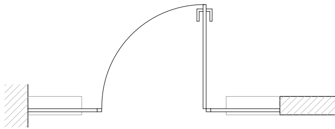
planta
