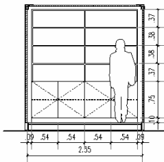
Corte B-B (Anchura de guardador/ director oficina)
