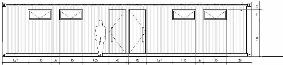
Corte B-B (Anchura de guardador/ director oficina)
