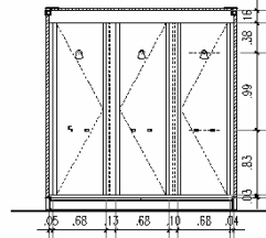
Corte C-C' (Boxes de ductos)
