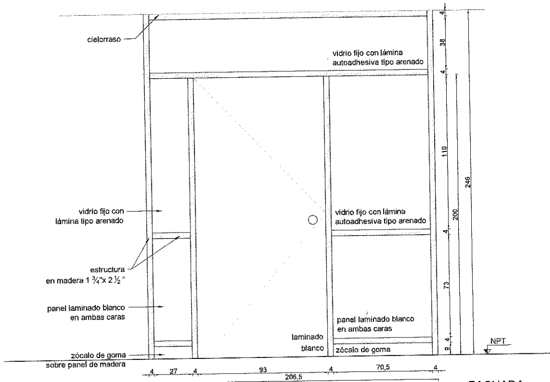
FACHADA
