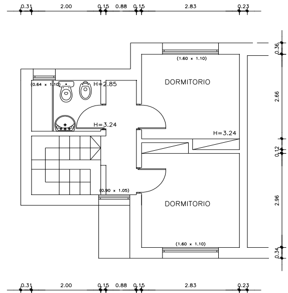
PLANTA ALTA
