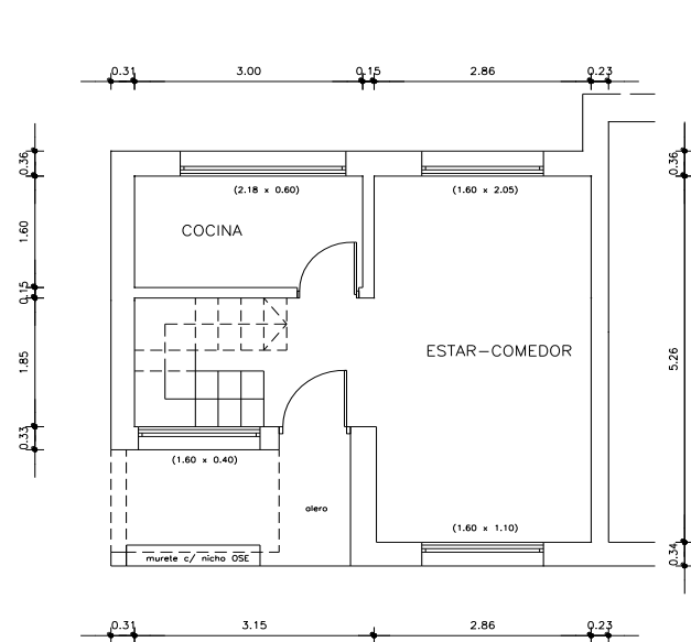
PLANTA BAJA.
