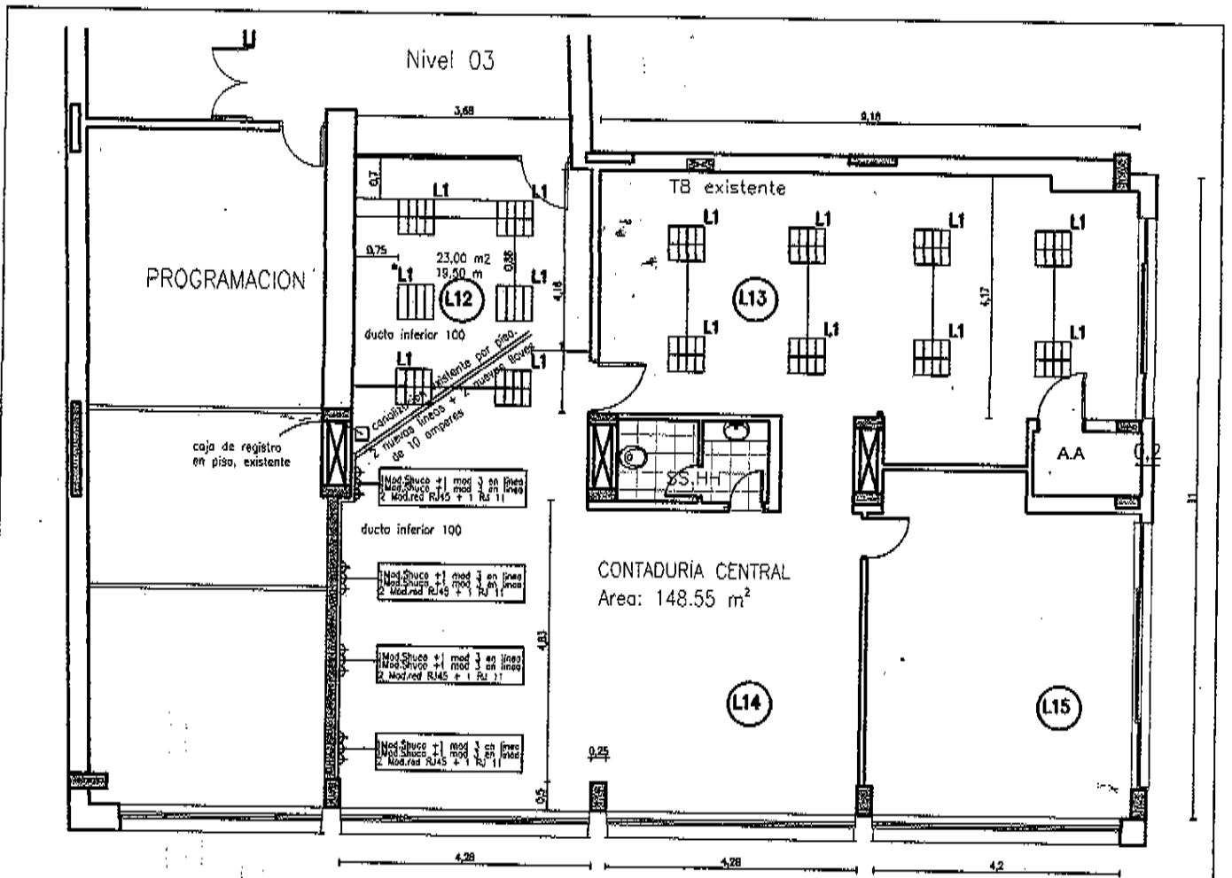
TERCER RISO: - CONTADURIA CENTRAL - INSTALACIÓN LUMÍNICA, ELÉCTRICA Y REDES. Área: 148.55 m 2
