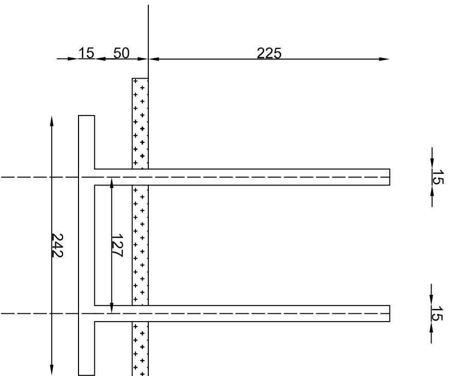
ALZADO
