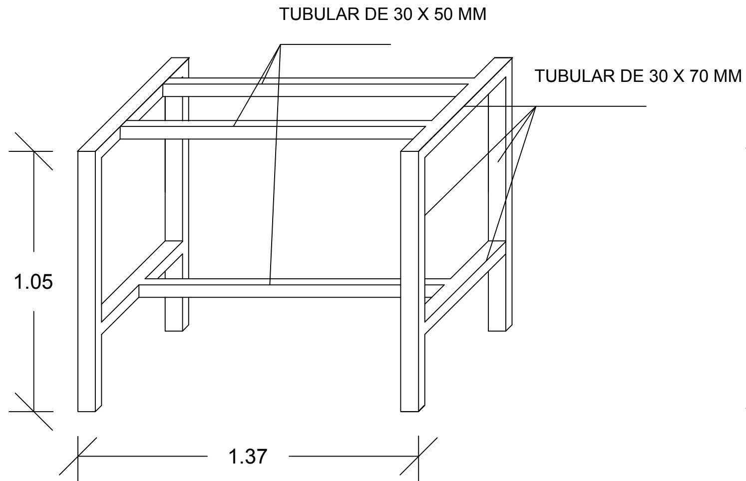
ESQUEMA BASE METÁLICA
