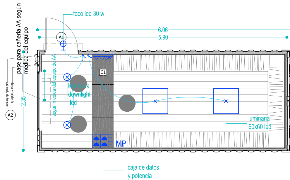
PLANTA Esc. 1/50
