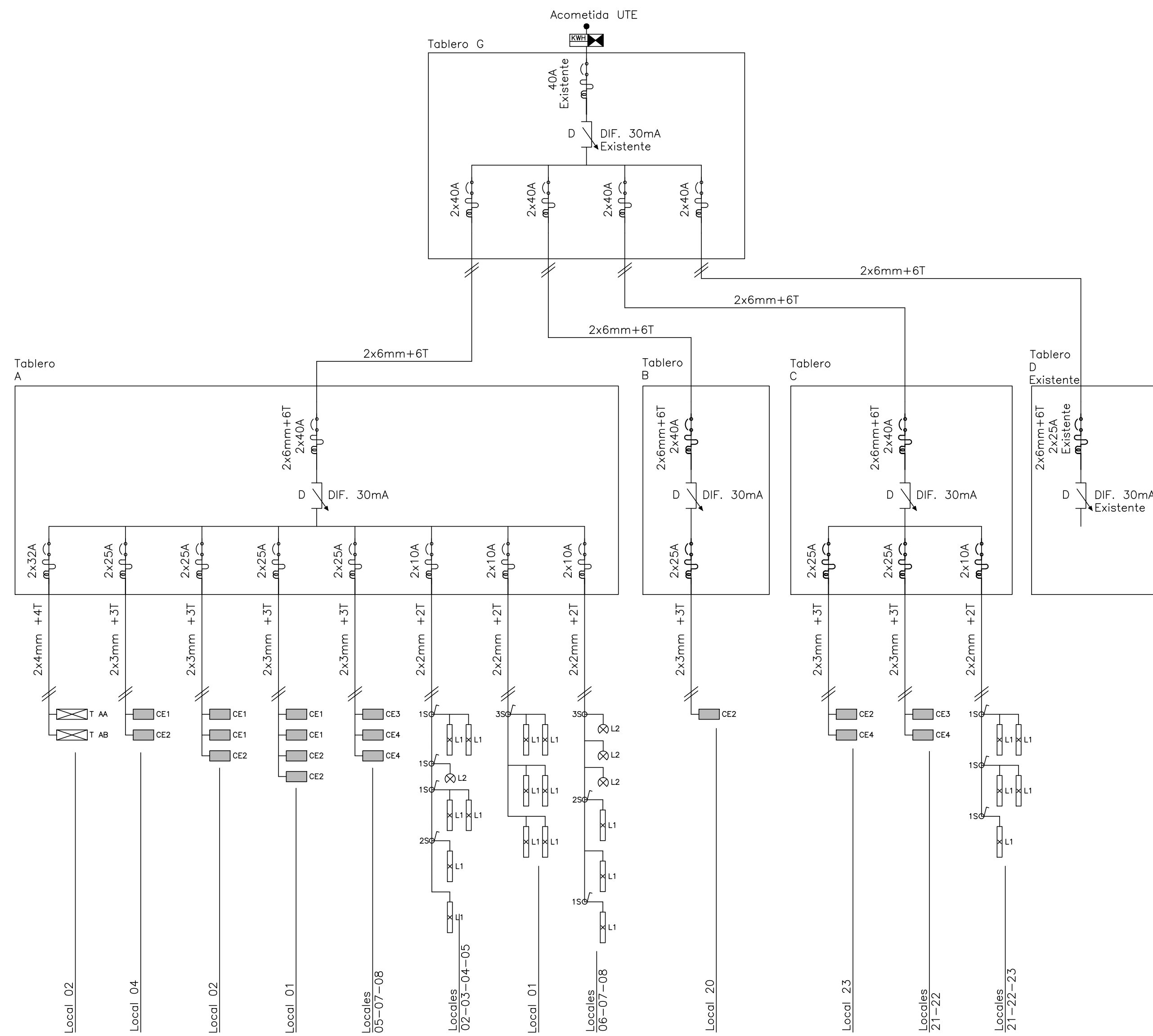
ESQUEMA UNIFILAR
