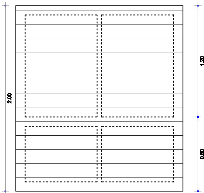
FACHADA
