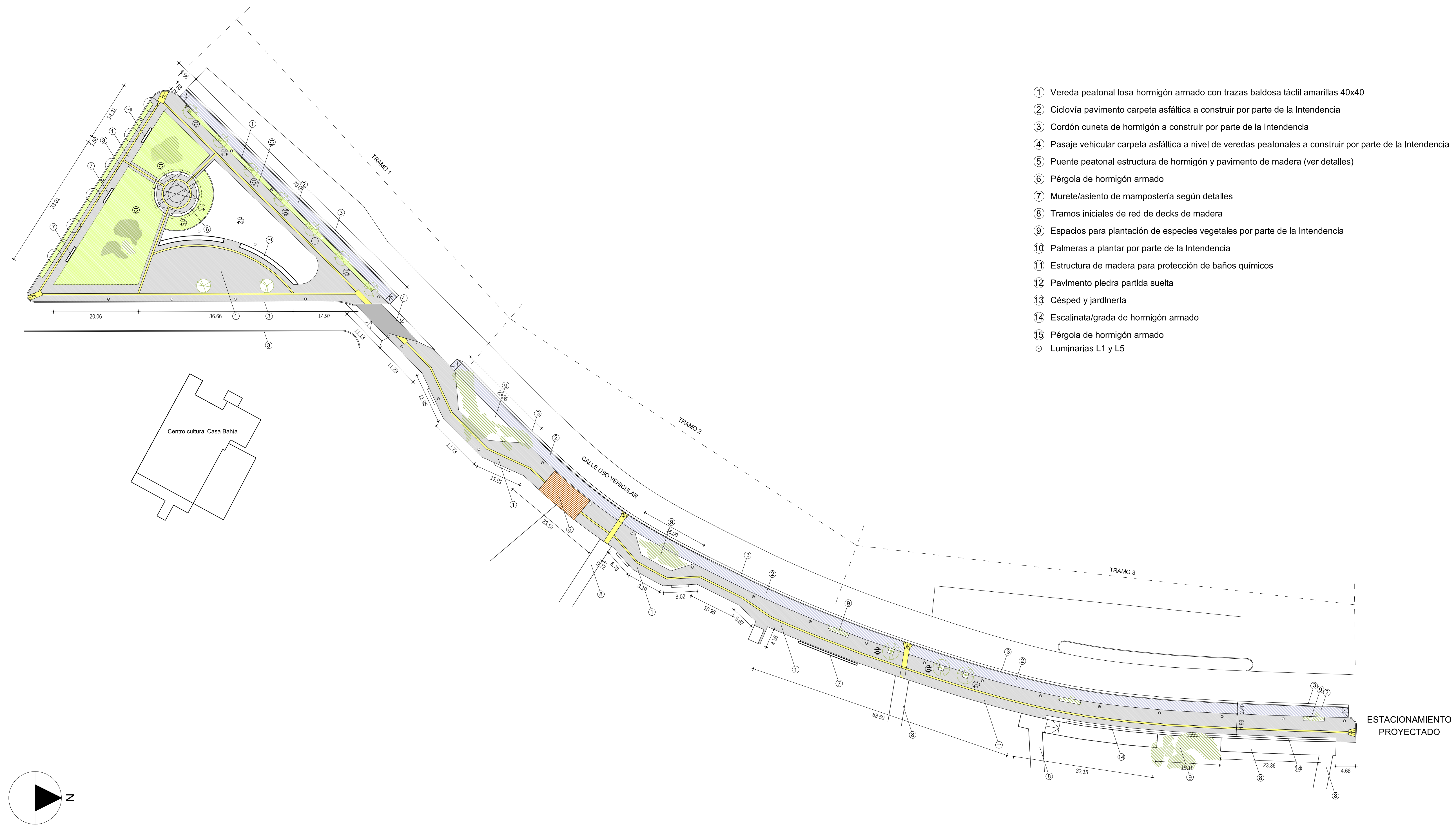
PLANTA GENERAL escala 1/500
