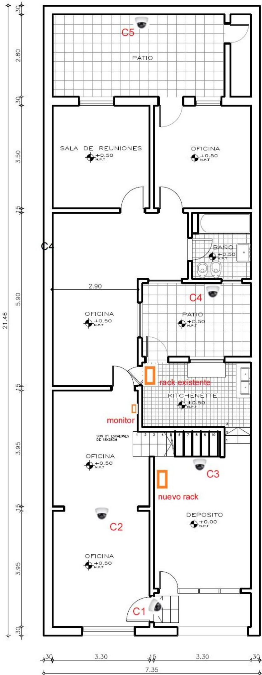
PLANTA BAJA – 87 m 2
