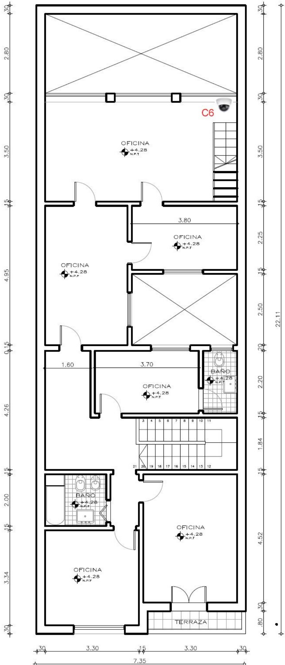
PLANTA ALTA - 57 M2
