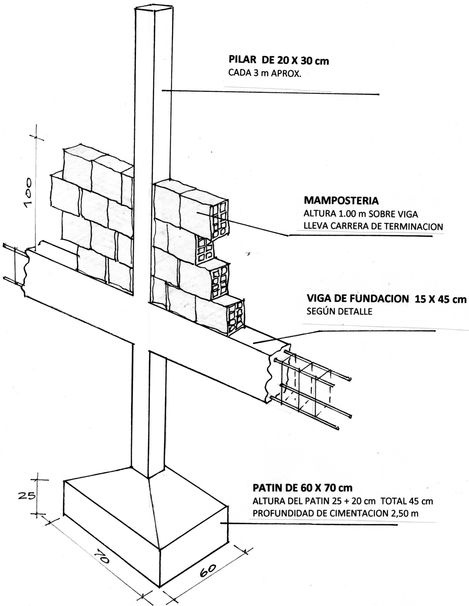
ESCUELA N° 88 CHUY DETALLE DE ESTRUCTURA DE MURETE
