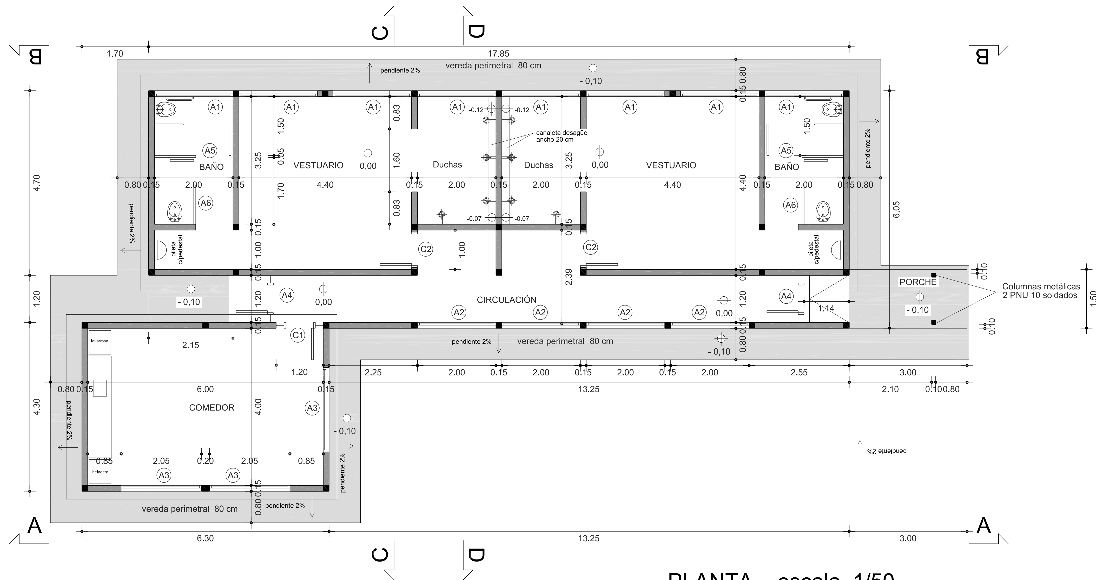
PLANTA escala 1/50
