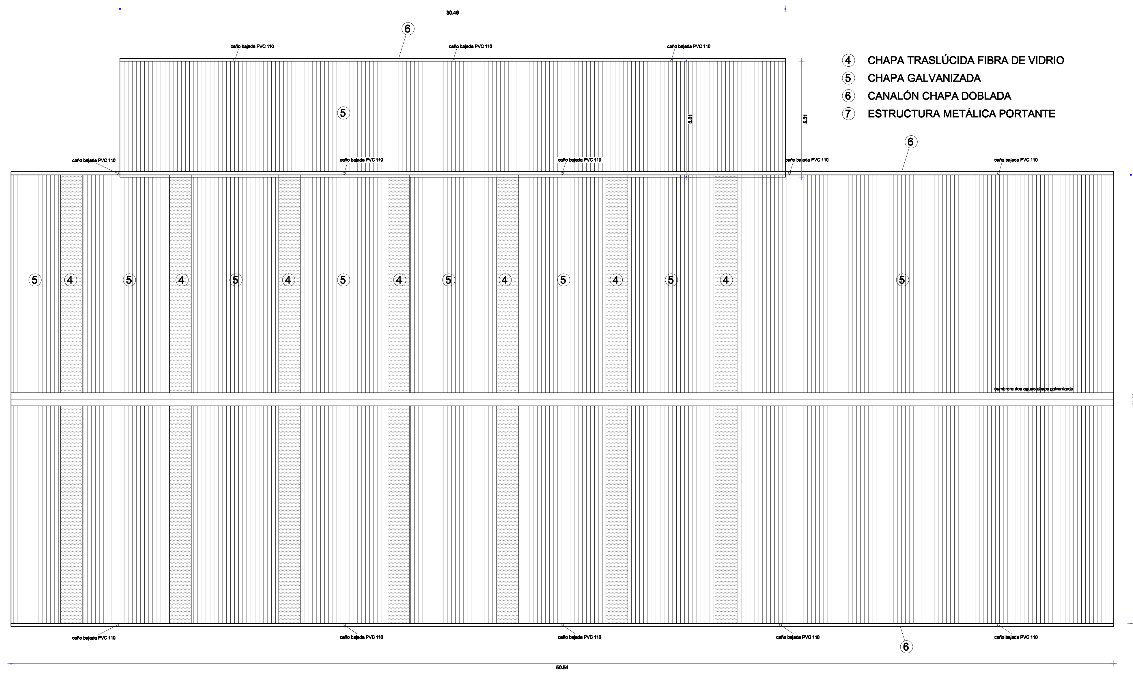
PLANTA CUBIERTA 1/100
