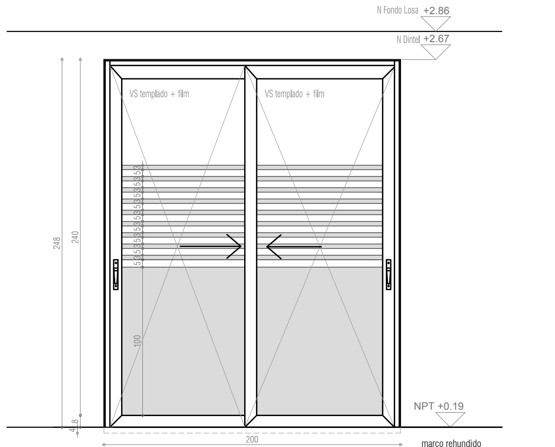
ALZADO
