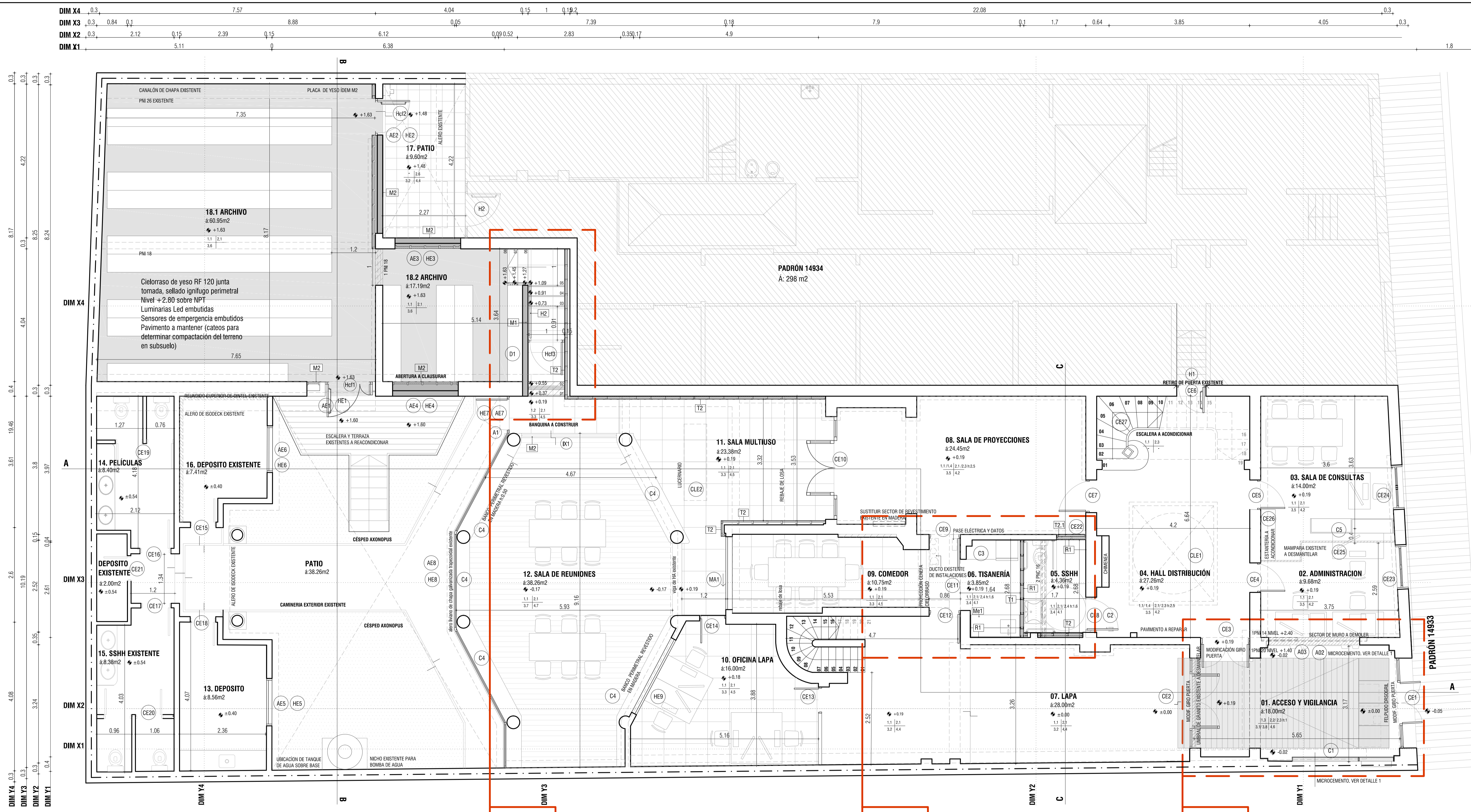
PLANTA BAJA ESC 1:50
