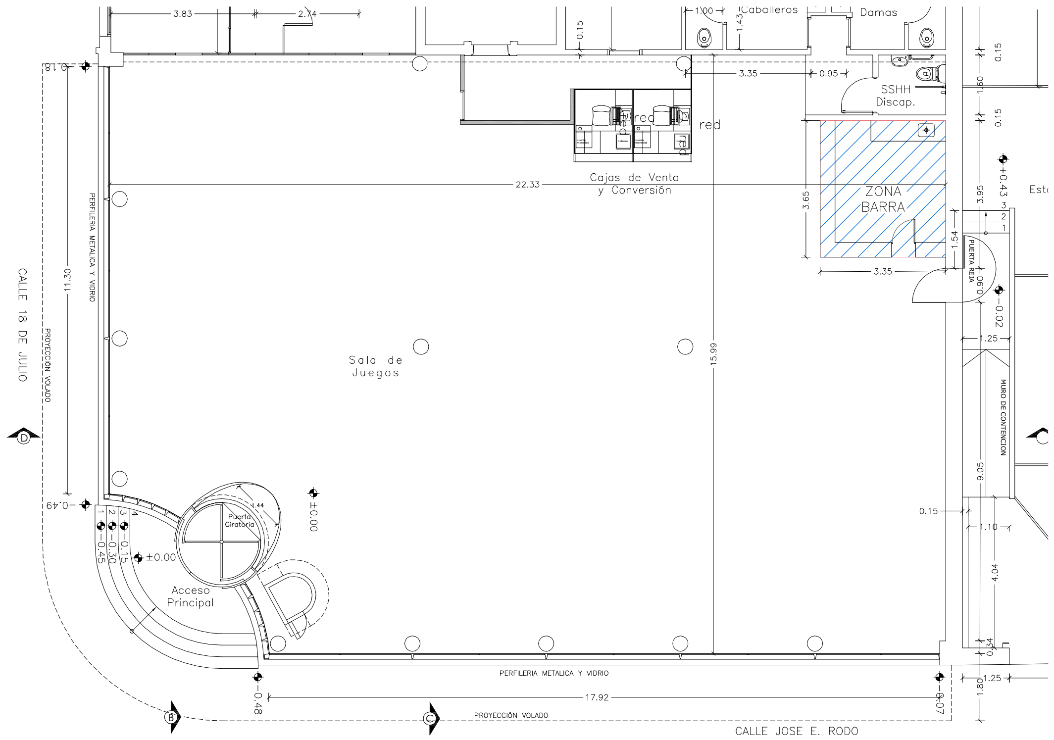
PLANTA BAJA (parcial)
