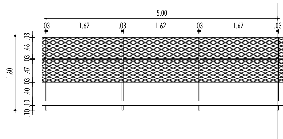
ALZADO FORONTAL Esc. 1:50
