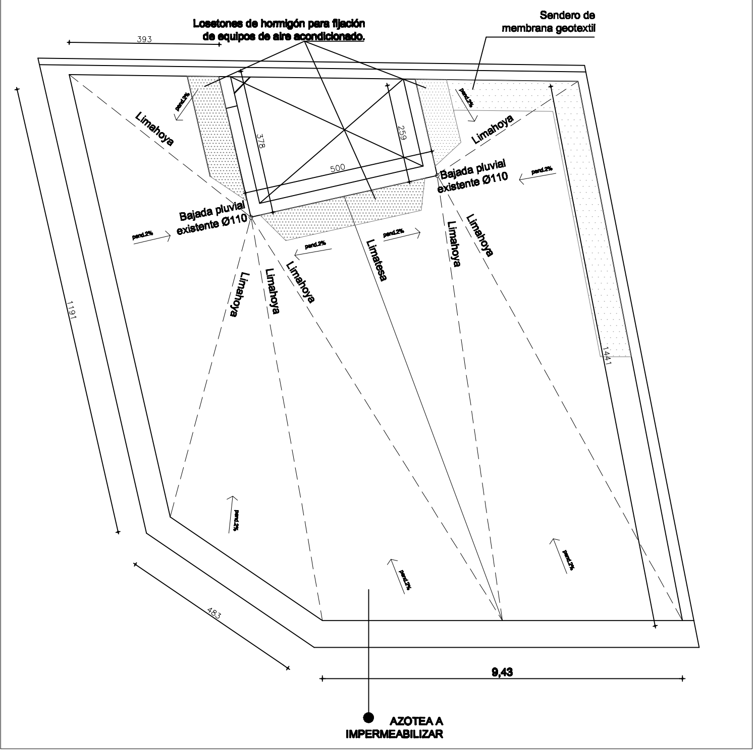
L1-PLANTA ESC.1:100
