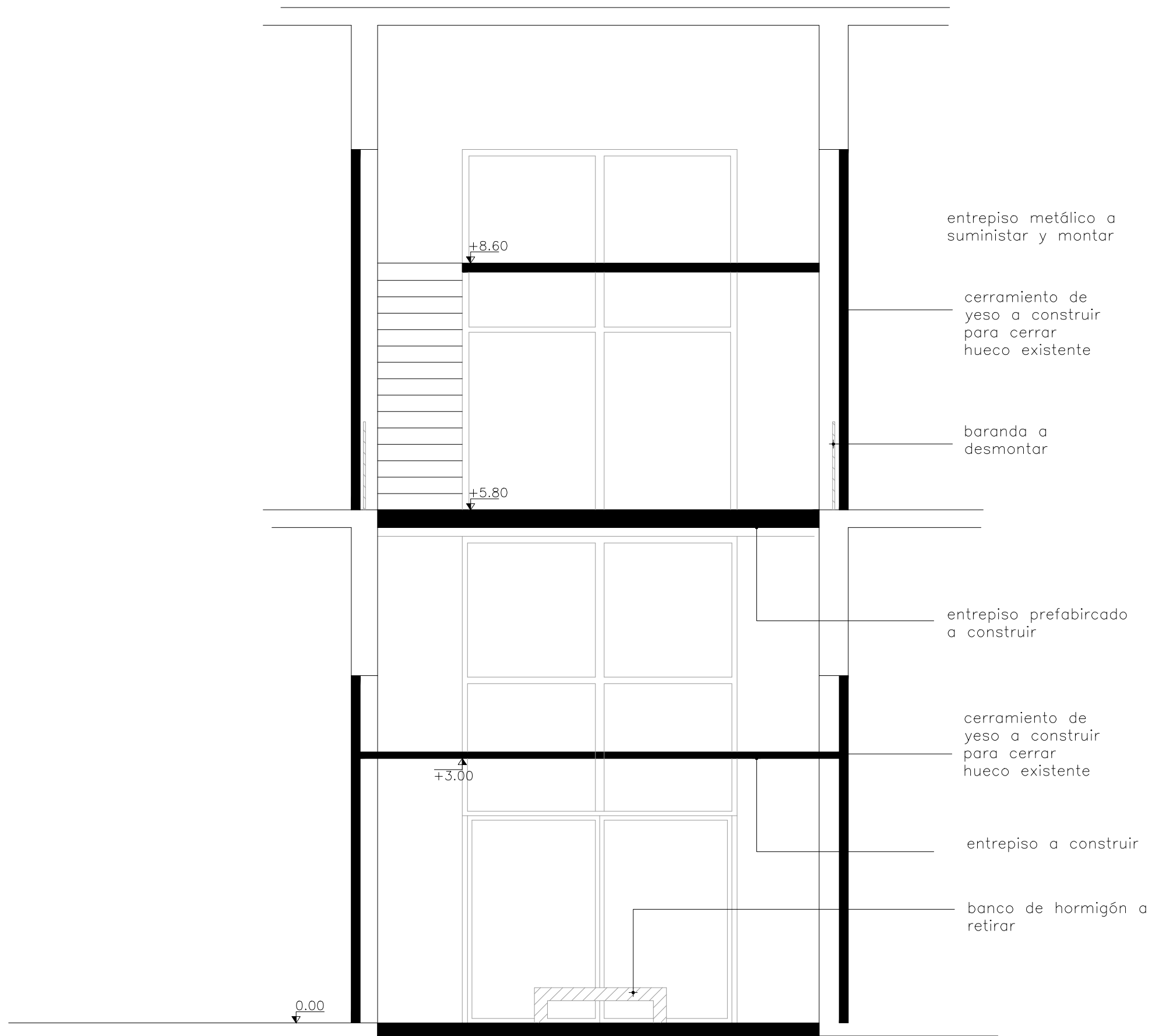
CORTE B-B
