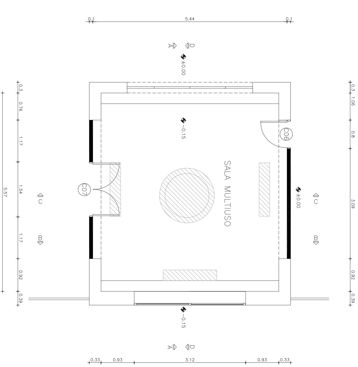
PLANTA BAJA
