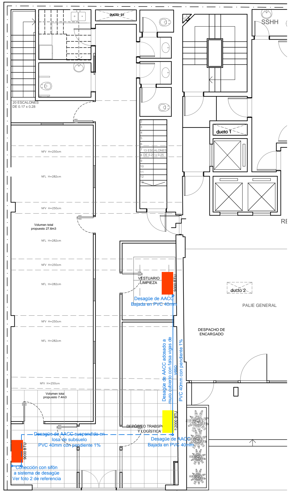
Planta baja Escala 1/75 - AACC
