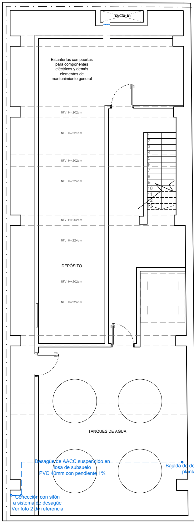
Planta subsuelo Escala 1/75 - AACC
