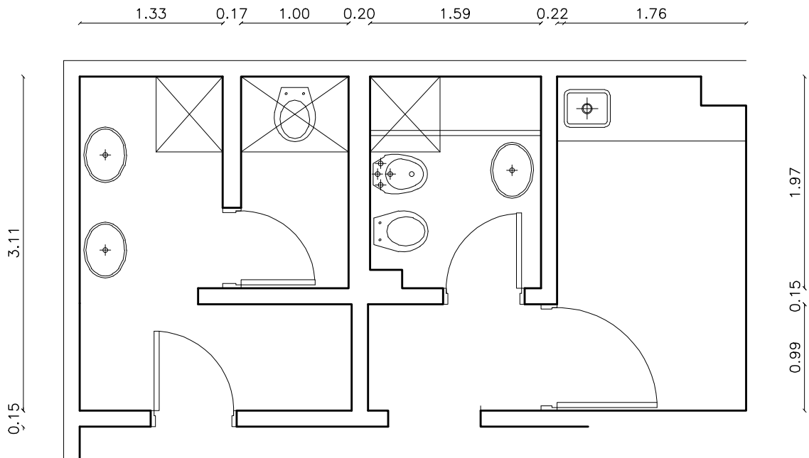
SITUACIÓN ACTUAL esc : 1/50
