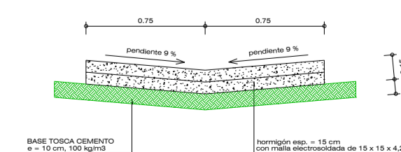
DETALLE BADEN DE HORMIGÓN Escala 30:1
