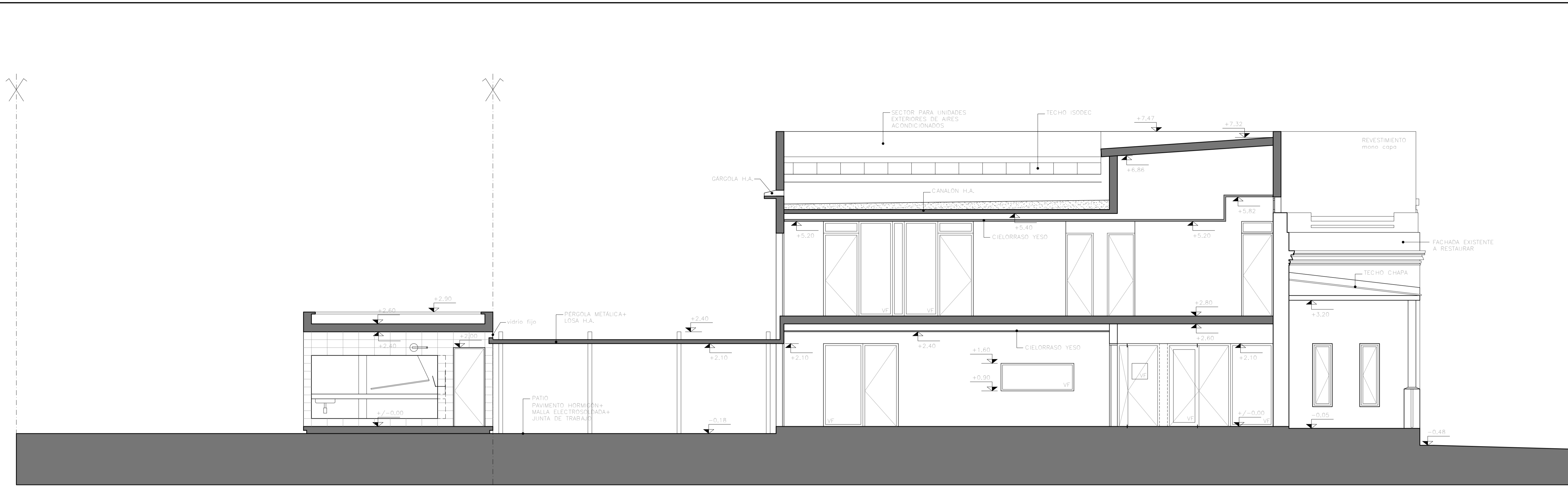
CORTE a-a Esc.: 1/50
