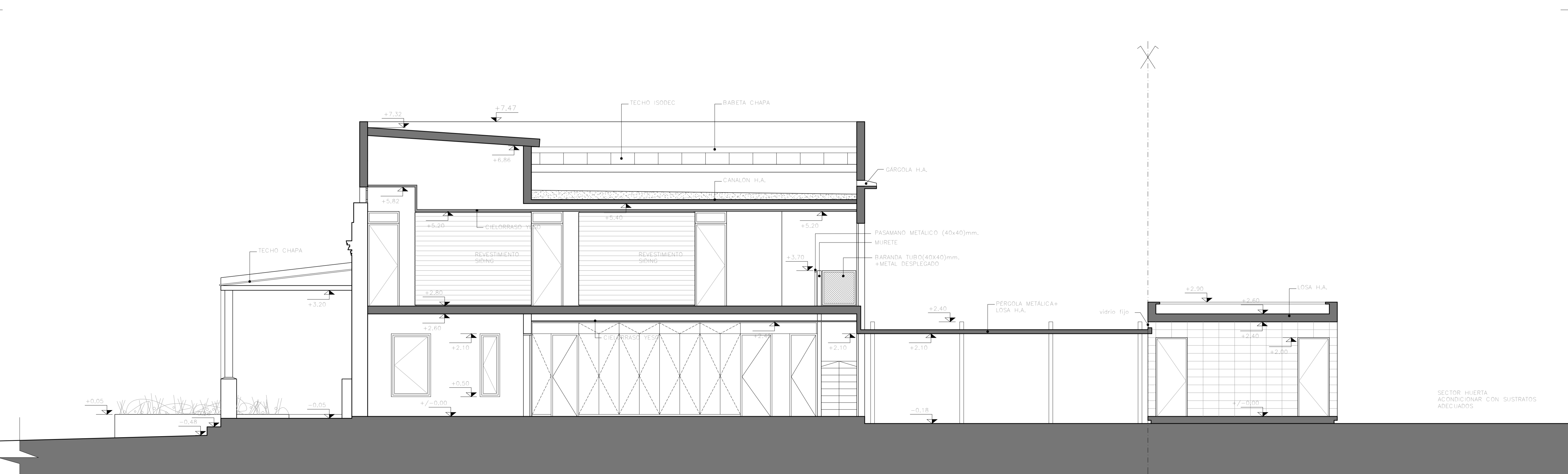
CORTE c-c Esc.: 1/50
