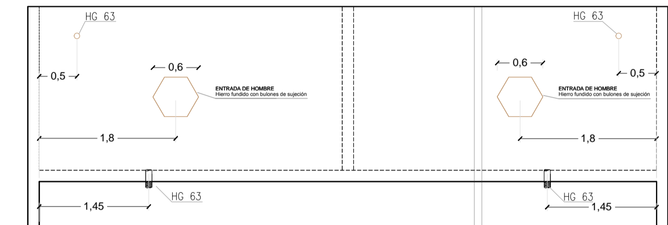
VISTA A-A
