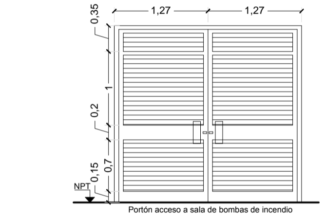
DETALLE ABERTURA 1/50
