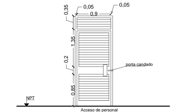
DETALLE ABERTURA 1/50
