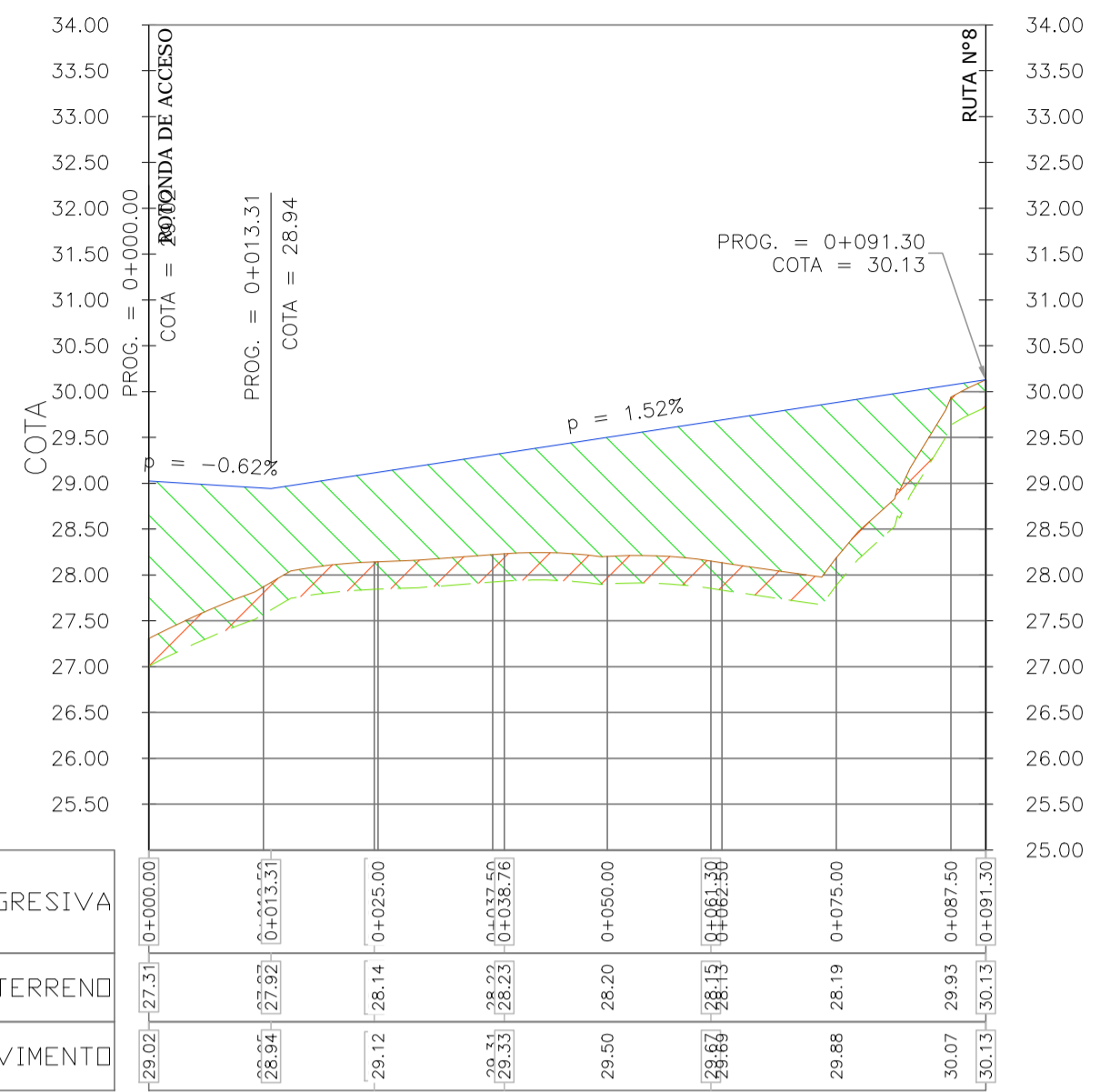
PERFIL LONGITUDINAL FVET - AVENIDA ACCESO - SALIDA Escala Horizontal: 1/750 Escala Vertical: 1/75
