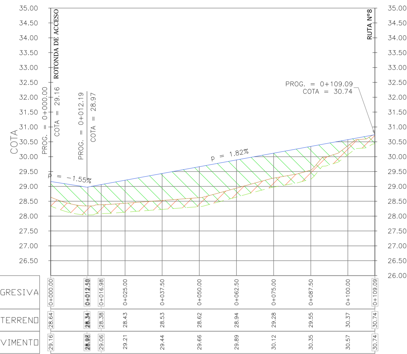
PERFIL LONGITUDINAL FVET - AVENIDA ACCESO - ENTRADA Escala Horizontal: 1/750 Escala Vertical: 1/75
