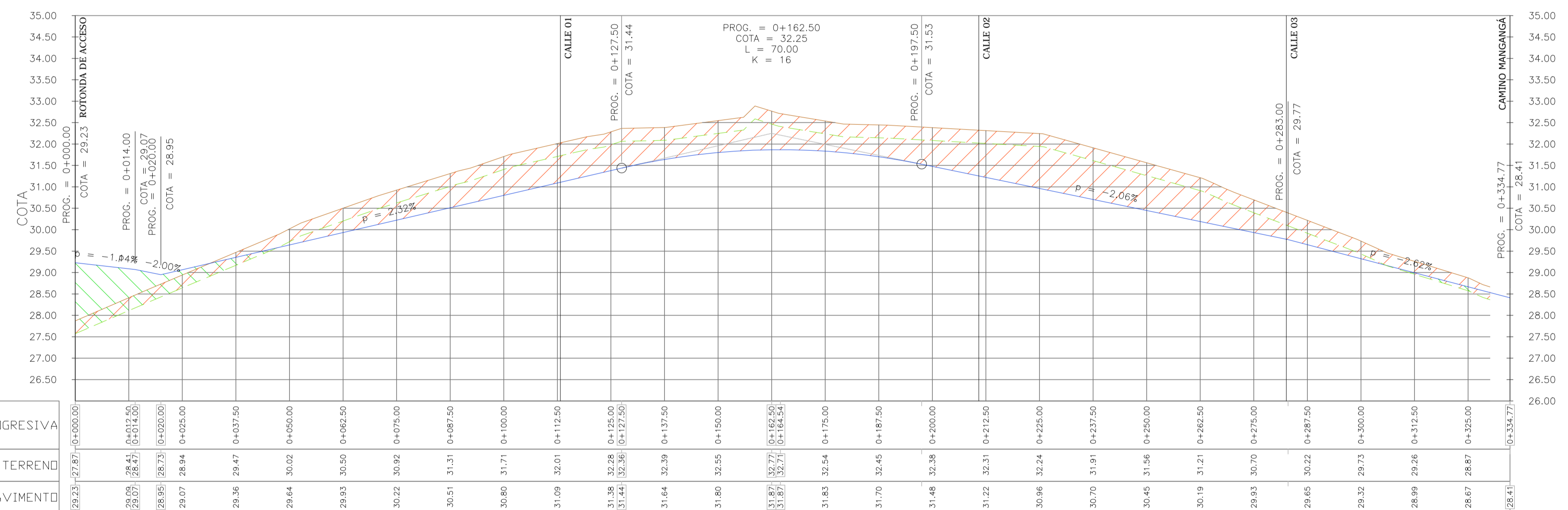
PERFIL LONGITUDINAL FVET - AVENIDA CENTRAL Escala Horizontal: 1/750 Escala Vertical: 1/75
