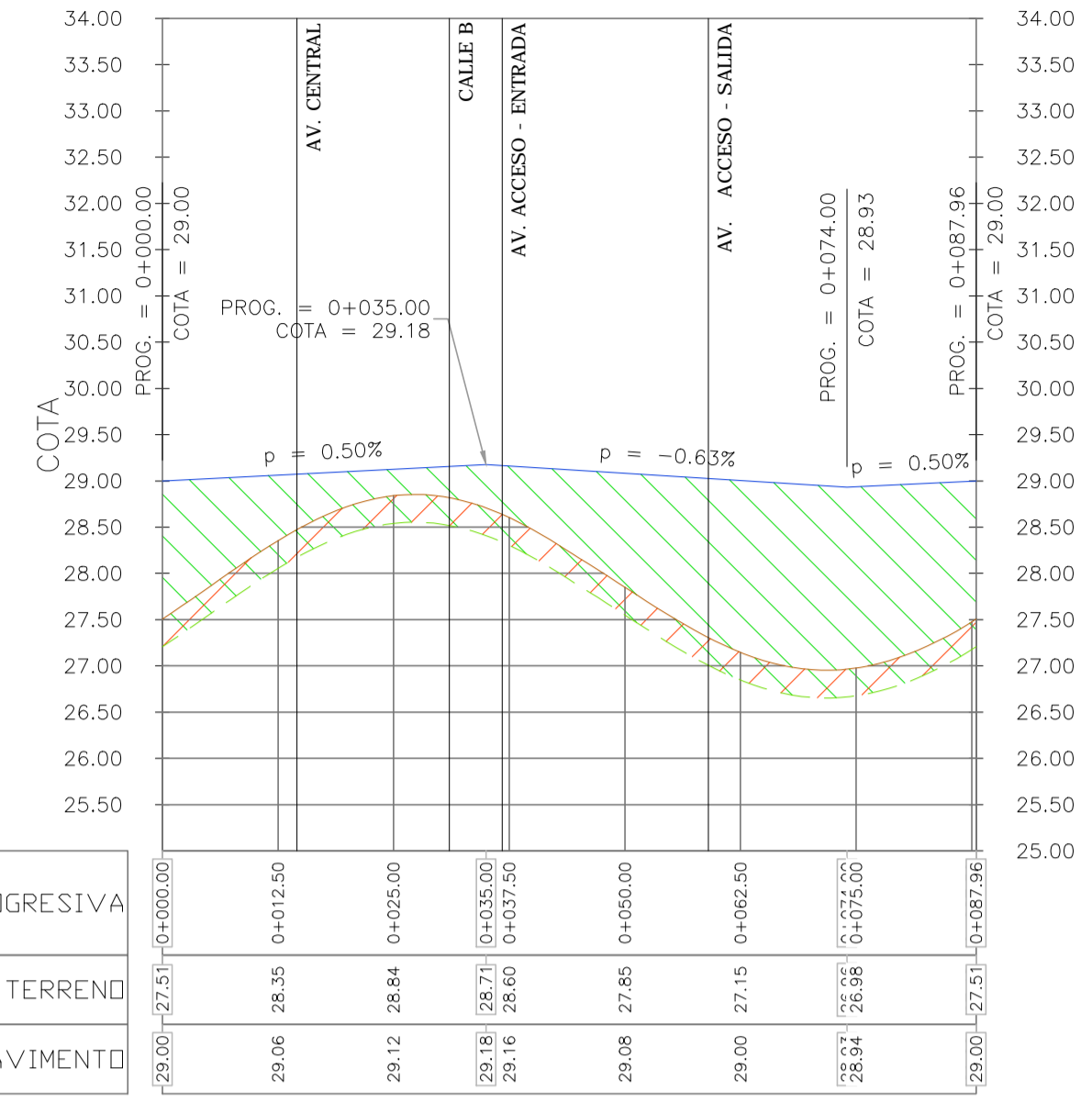
PERFIL LONGITUDINAL FVET - ROTONDA Escala Horizontal: 1/750 Escala Vertical: 1/75
