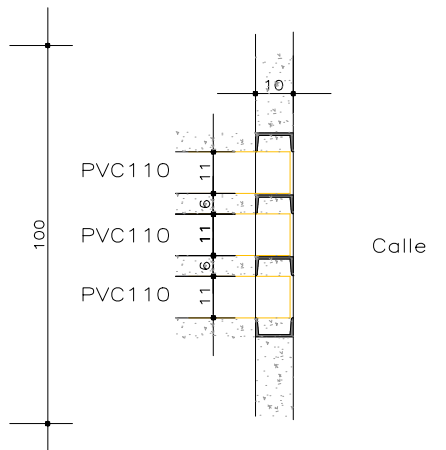
Salida de Pluvial Lab. Mecanica planta esc.1/20
