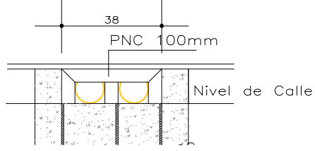
Salidas de Pluviales vista frontal esc. 1/20
