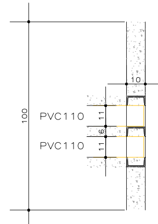
Salidas de Pluviales planta esc. 1/20
