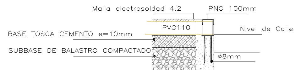
Salidas de Pluviales vista corte esc. 1/20
