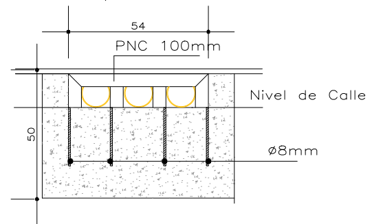
Salidas de Pluviales vista lab. Mecanica frontal esc. 1/20
