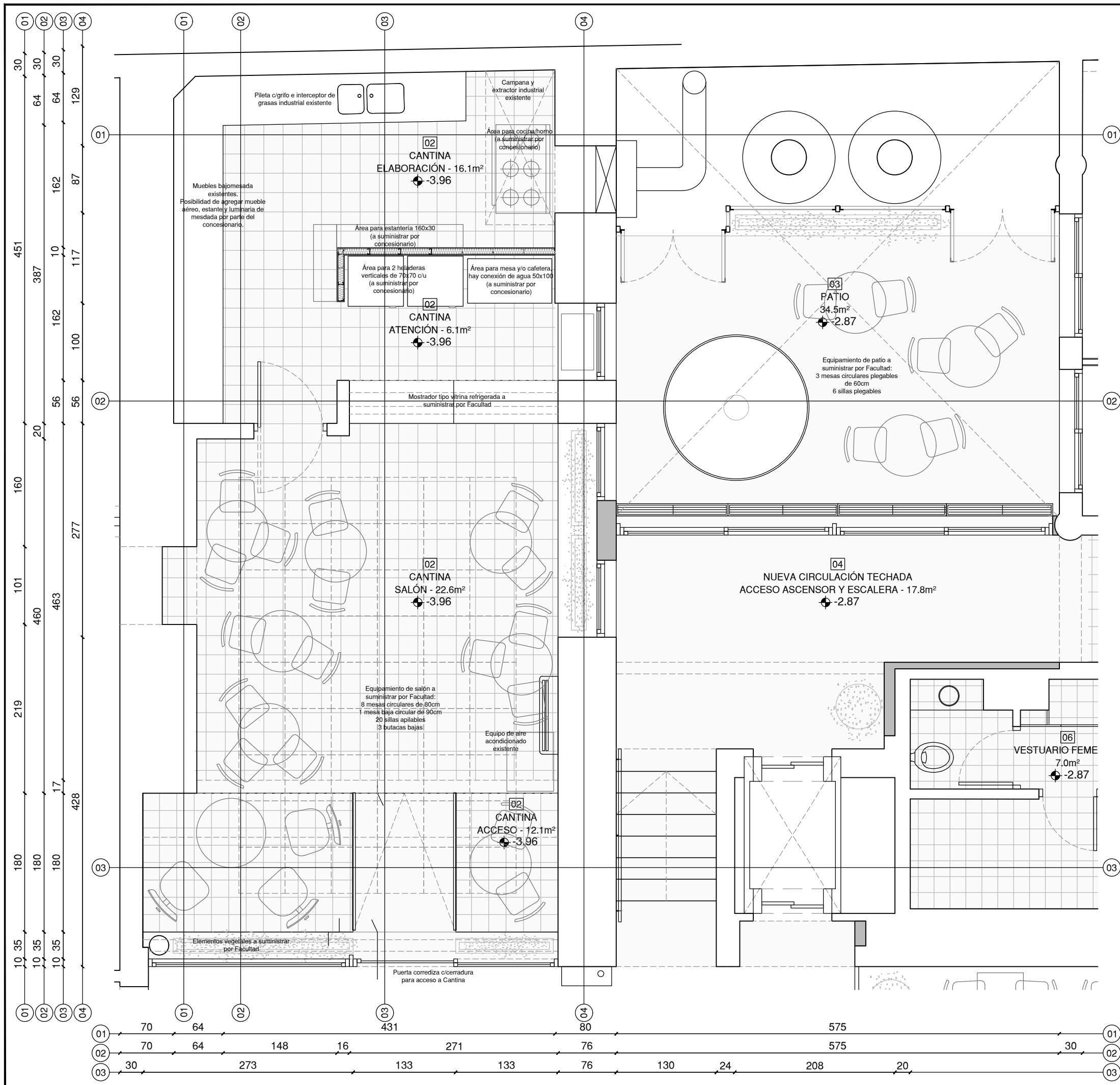
PLANTA SUBSUELO SECTOR CANTINA Y PATIO ESC 1/50
