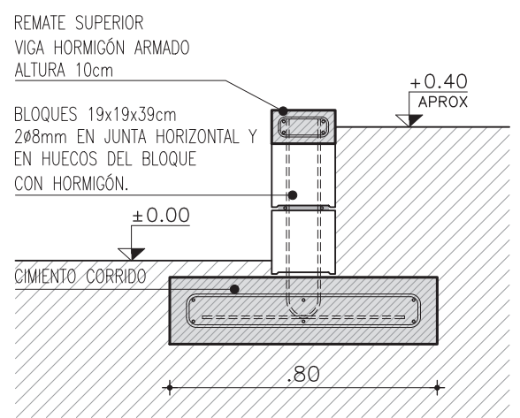
DETALLE MURO DE CONTENCIÓN
