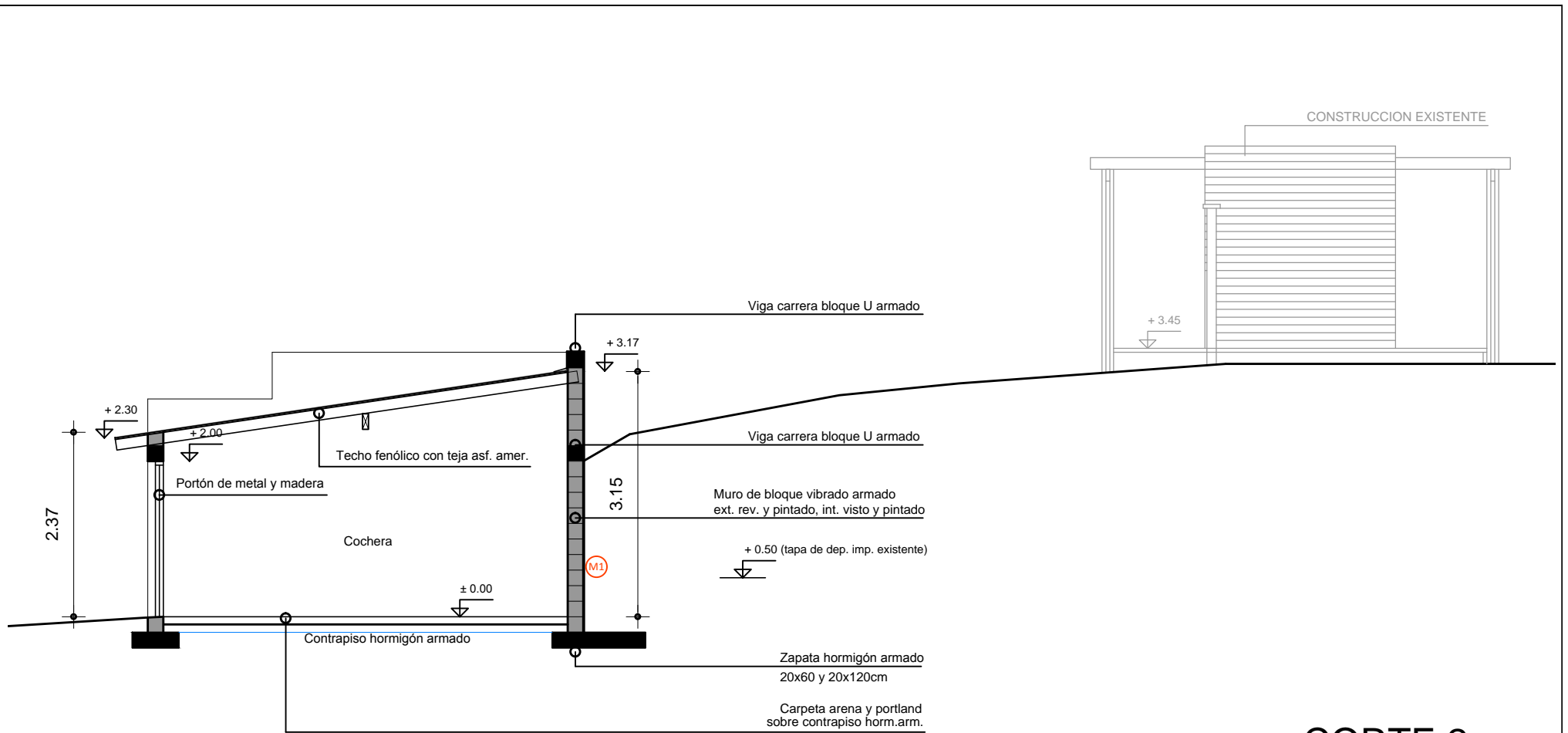
CORTE 2 escala 1:75
