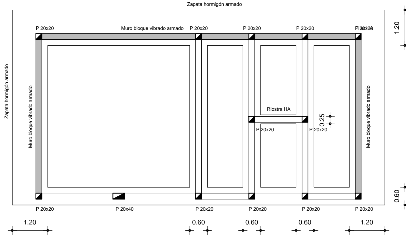
PLANTA FUNDACION escala 1:75
